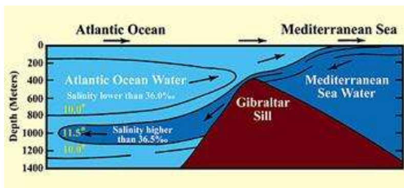
Figura 1. Marea Mediterană atunci când intră în Atlantic prin strâmtoarea Gibraltar cu apa ei caldă, sărată și mai puțin densă din cauza barierei care face diferența dintre ele. Temperatura este în Celsius. (Marine Geology, Keunen, p.43)
